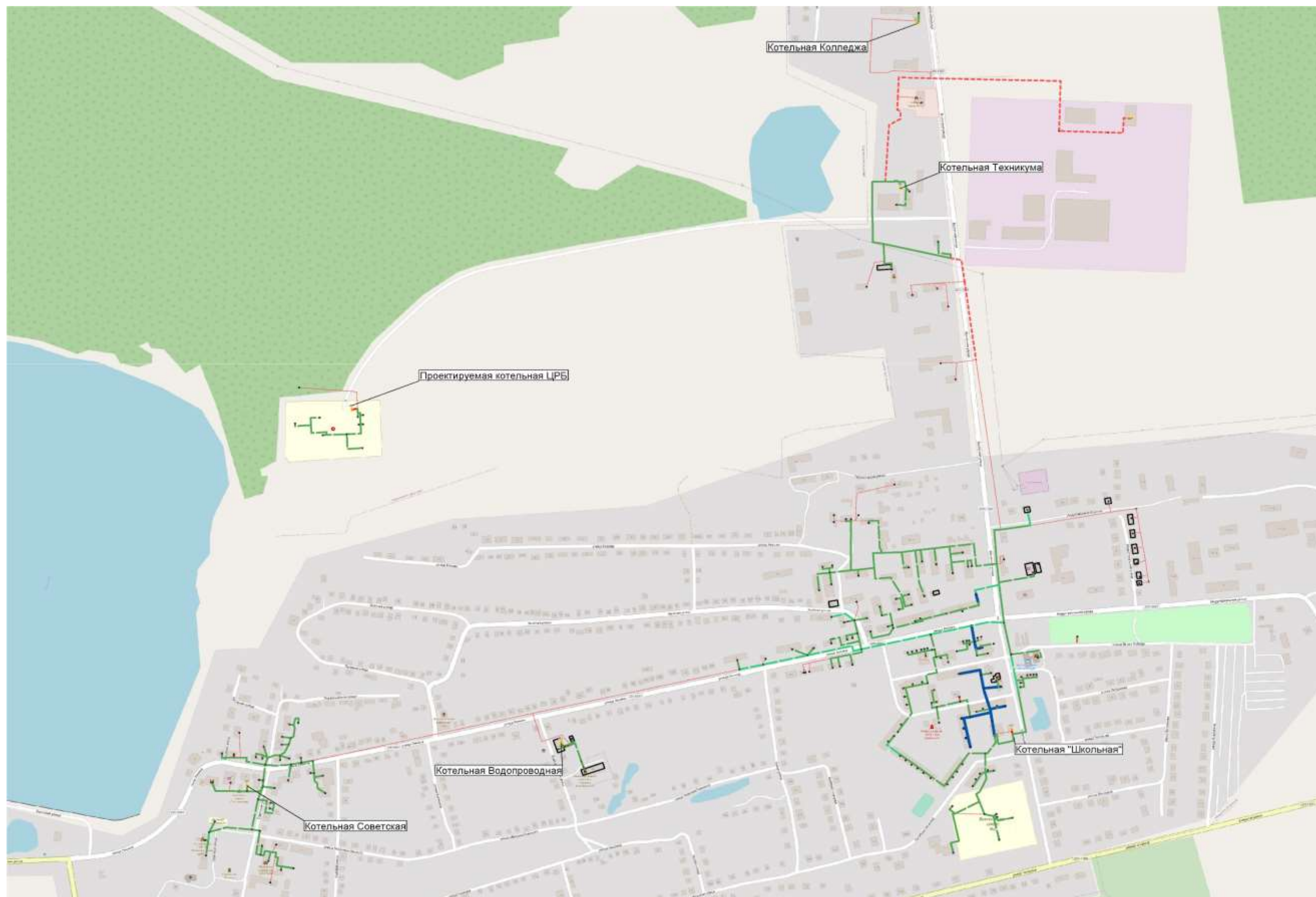
Рисунок 14.1. Ситуационный план источников теплоснабжения р.п. Вознесенское
